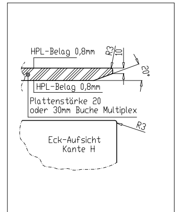
Kante H Tischplatte 20 mm stark, Trägermaterial Buche-Multiplex, R 3 mm nach unten abgeschrägt
