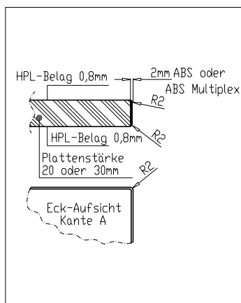
Kante A Tischplatte 20 oder 30 mm stark, mit 2 mm ABS-Anleimer in verschiedenen Farben
