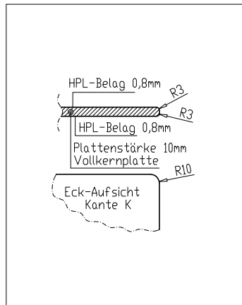
Kante K Tischplatte 10 mm stark, Vollkernplatte Radius oben und unten 3 mm
