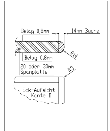
Kante D Tischplatte 30 mm stark, mit Massivholz-Anleimer 30 x 14 mm, Ecken leicht gerundet, ballig gefräst
