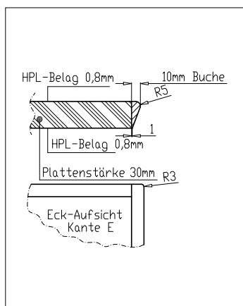
Kante E Tischplatte 30 mm stark, mit Massivholz-Anleimer, 30 x 10 mm R 5 mm nach unten abgeschrägt
