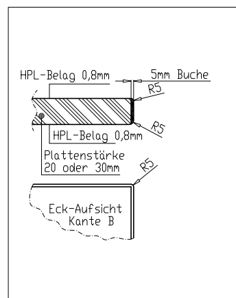
Kante B Tischplatte 20 oder 30 mm stark, mit 5 mm Massivholz-Anleimer
