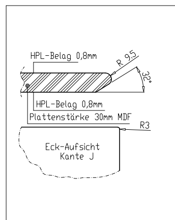
Kante J Tischplatte 30 mm stark, Trägermaterial MDF, R 9,5 mm nach unten abgeschrägt
