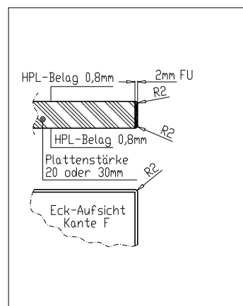
Kante F Tischplatte 20 oder 30 mm stark, mit 2 mm Furnier-Anleimer
